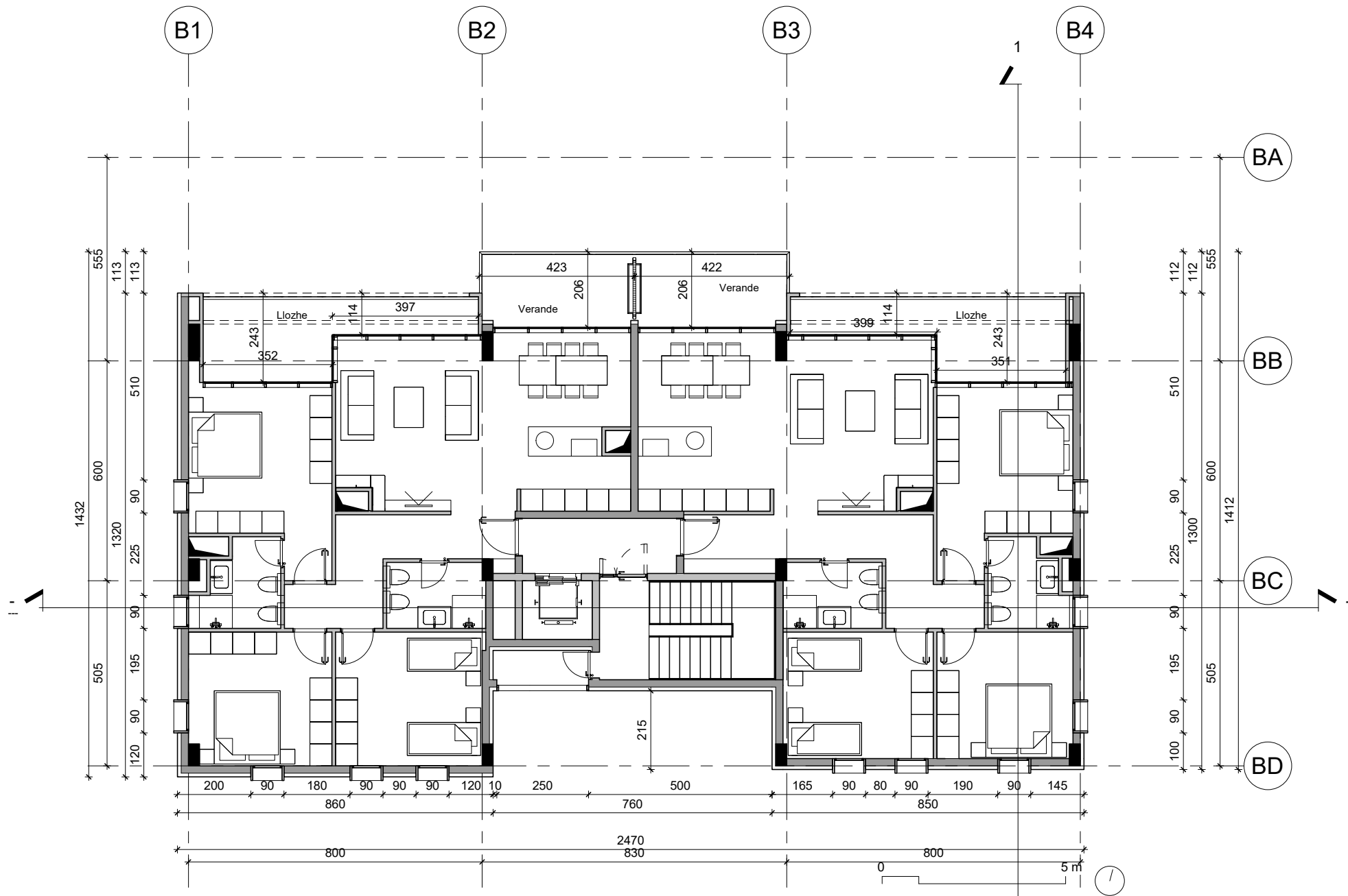
objekt B - plan i katit 1
