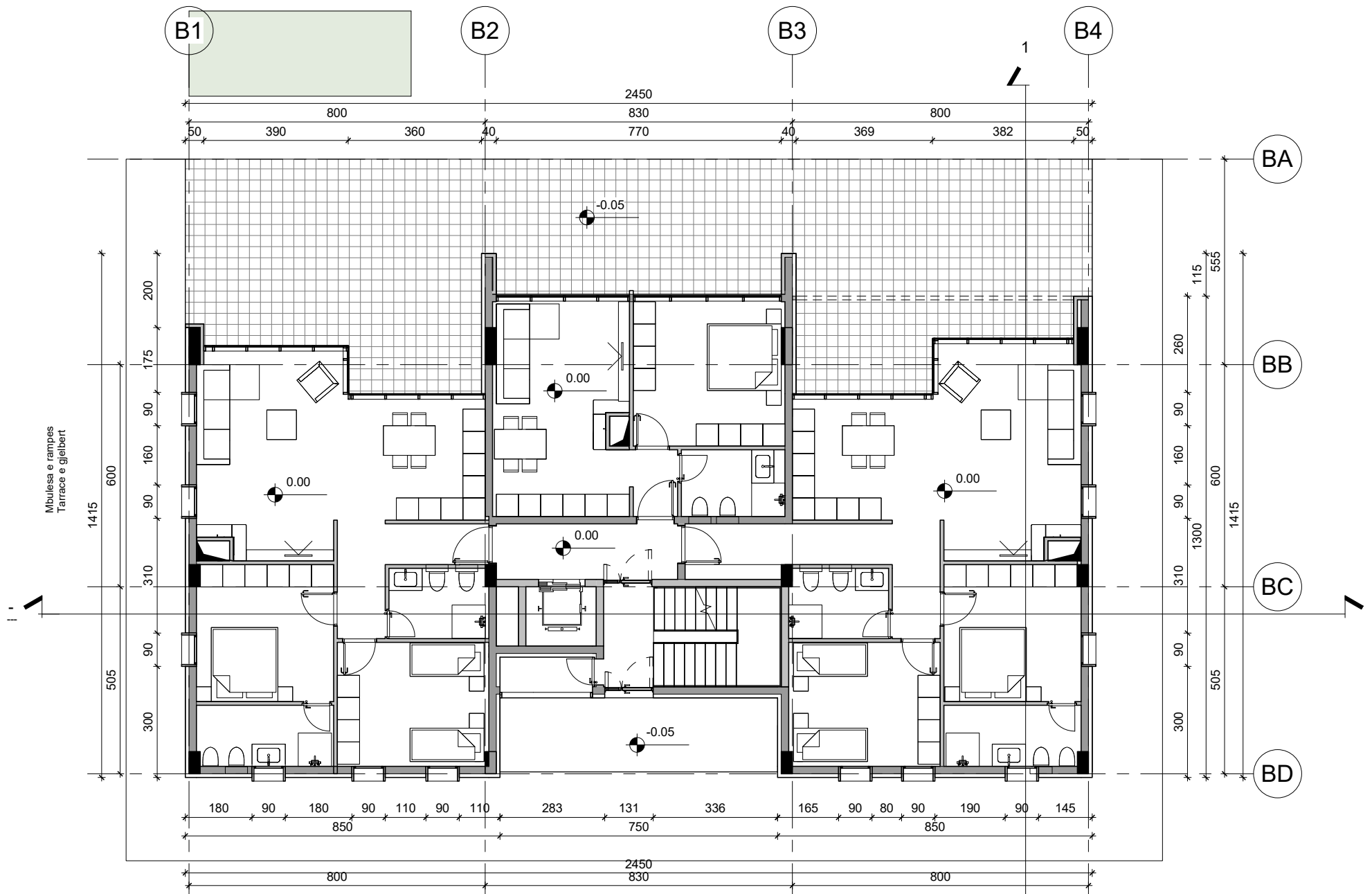
objekti B - plan i katit 0
