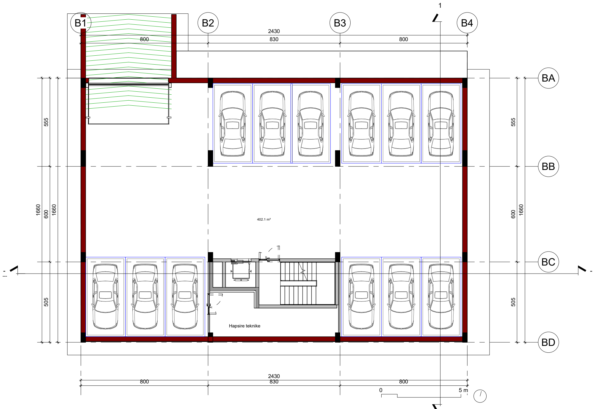
objekt B - plan i katit nentoke
